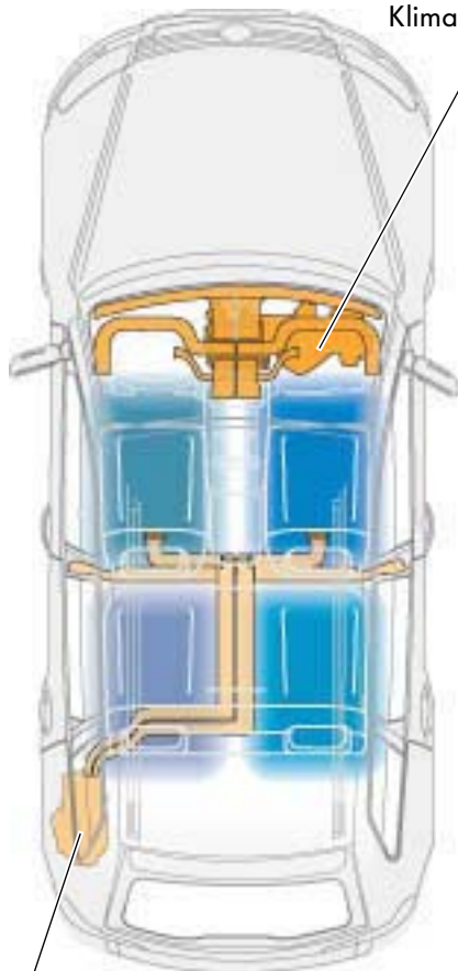
Klimagerät hinten
